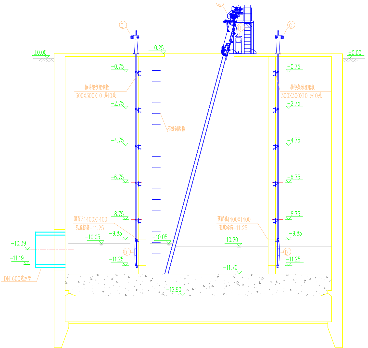
1-1剖面图 1:100
